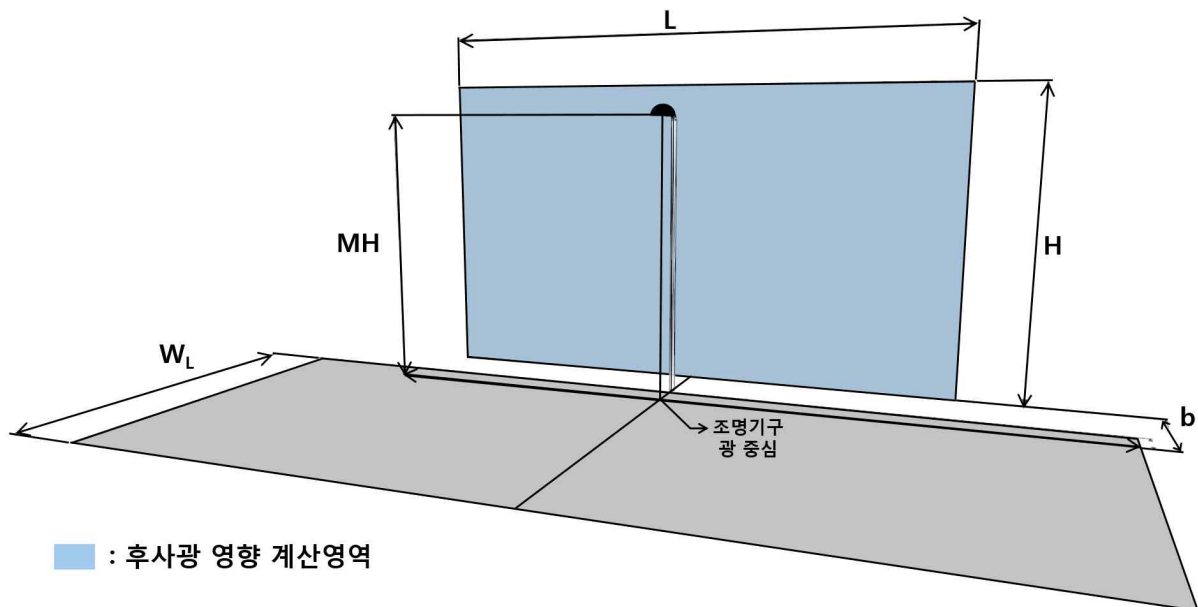
(2) 후사광 영향에 대한 조도 계산 영역
