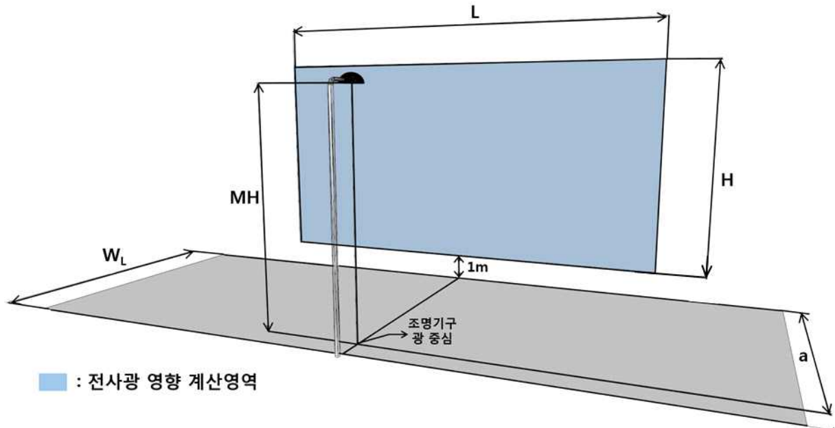
(1) 전사광 영향에 대한 조도 계산 영역
